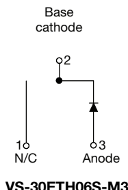
D²PAK (TO-263AB)
