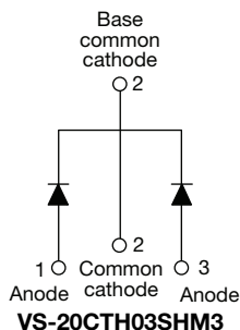
D²PAK (TO-263AB)
