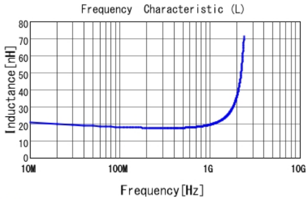
■ LQG15HN18NJ02 L
