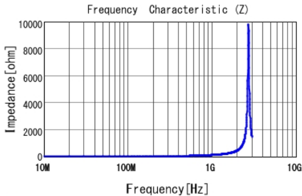
■ LQG15HN18NJ02 |Z|
