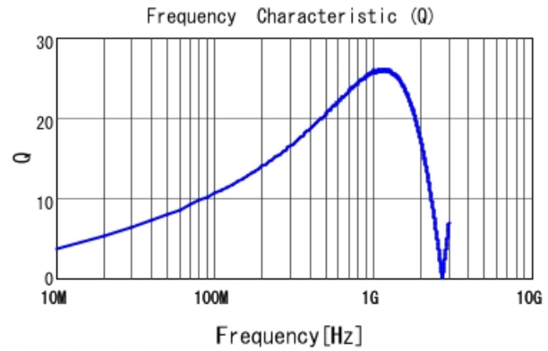
■ LQG15HN18NJ02 Q
