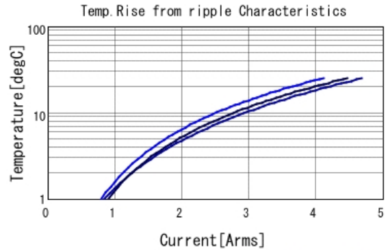
KRM55WR71J226MH01 Temp. rise ■ 50kHz ■ 100kHz ■ 300kHz
