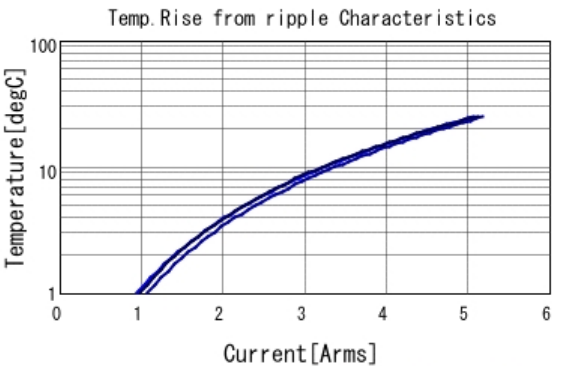
KRM55WR71H336MH01 Temp. rise ■ 50kHz ■ 100kHz ■ 300kHz
