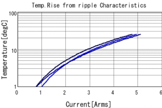
KRM55TR71H226MH01 Temp. rise ■ 50kHz ■ 100kHz ■ 300kHz
