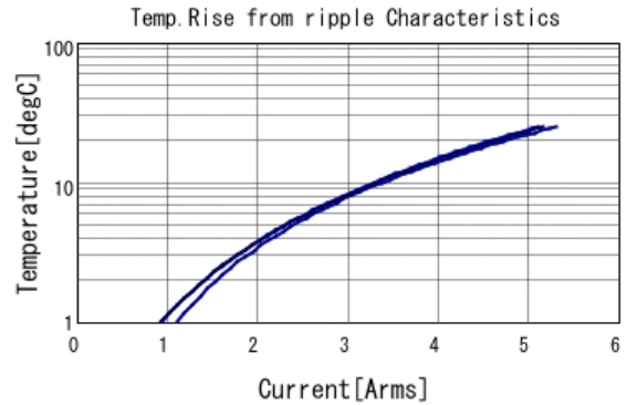
KRM55TR71E336MH01 Temp. rise ■ 50kHz ■ 100kHz ■ 300kHz
