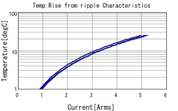
KRM55QR71E336KH01 Temp. rise ■ 50kHz ■ 100kHz ■ 300kHz
