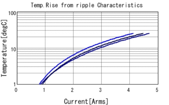
KCM55WR72A226MH01 Temp. rise ■ 50kHz ■ 100kHz ■ 300kHz
