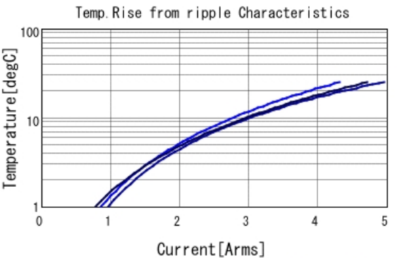
KCM55WR72A156MH01 Temp. rise ■ 50kHz ■ 100kHz ■ 300kHz
