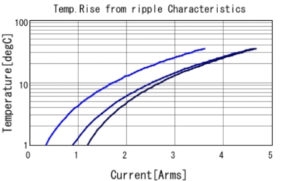
GRT155C80E106ME13 Temp. rise ■ 80kHz ■ 400kHz ■ 800kHz
