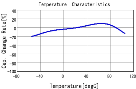
■ GRT155C80E106ME13 C-Temp. capchange, DCO. 0V, ACO. 05Vr
