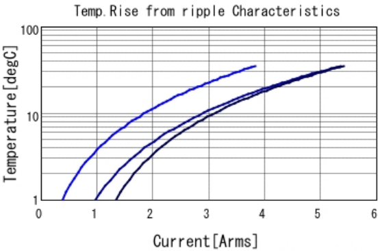
GRM21BR70J106KA73 Temp. rise ■ 80kHz ■ 400kHz ■ 800kHz
