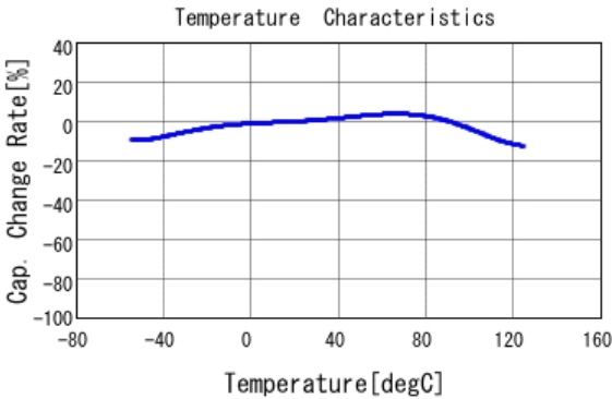
■ GRM21BR70J106KA73 C-Temp. capchange, DCO. 0V, ACO. 35Vr
