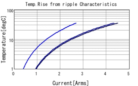
GRM188C70J225KE20 Temp. rise ■ 100kHz ■ 500kHz ■ 1MHz
