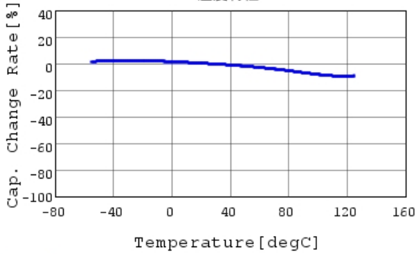
温度特性
