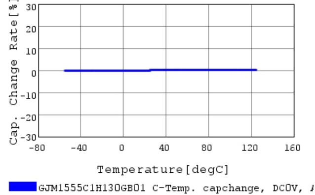
温度特性
