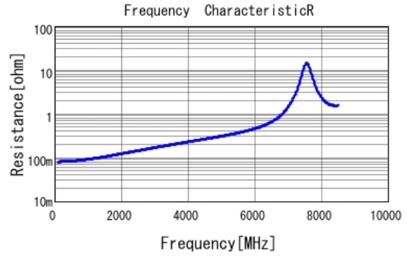
■ GCQ1555C1H8R4WB01 R DC0V, 25degC
