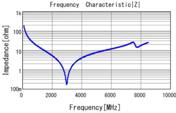
■ GCQ1555C1H8R4WB01 |Z| DC0V, 25degC
