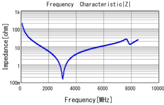
■ GCQ1555C1H8R1CB01 |Z| DCOV, 25degC
