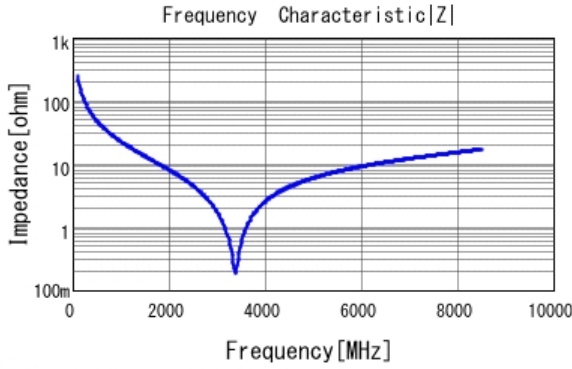
■ GCQ1555C1H6R4DB01 |Z| DC0V, 25degC
