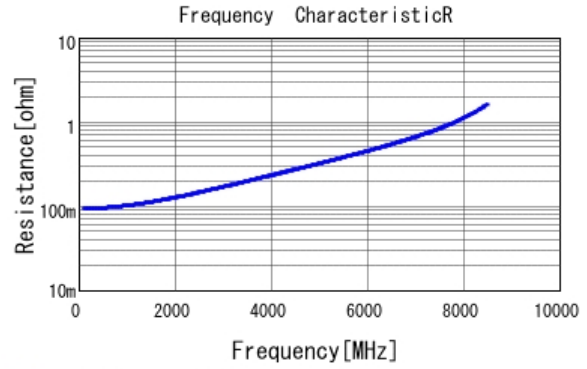
■ GCQ1555C1H6R4DB01 R DC0V, 25degC
