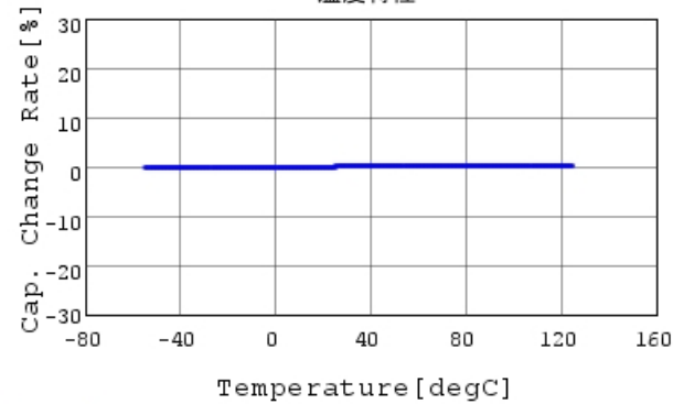
温度特性
