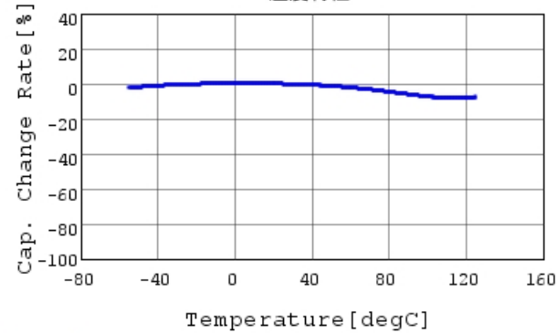
温度特性
