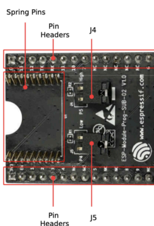
Fig. 2: ESP-Module-Prog-SUB-02 - Front
