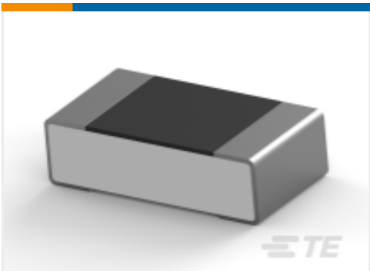
TE Part # 2176370-8 RQ 0603 511R 0.1% 10PPM 5K RL
