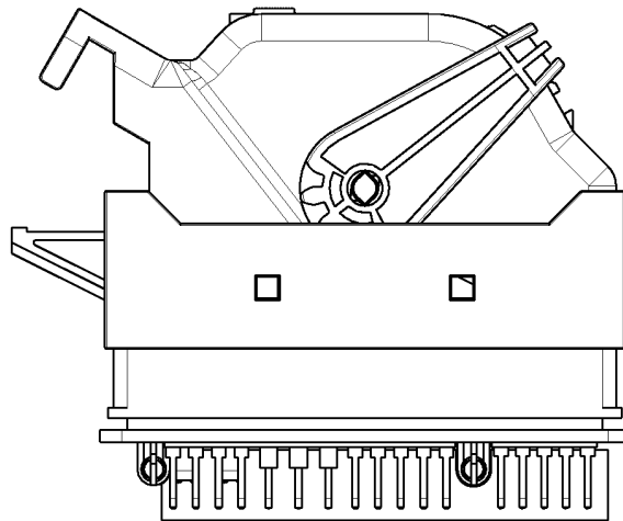
Slide open / Schieber offen Figure 12 / Abbildung 12
